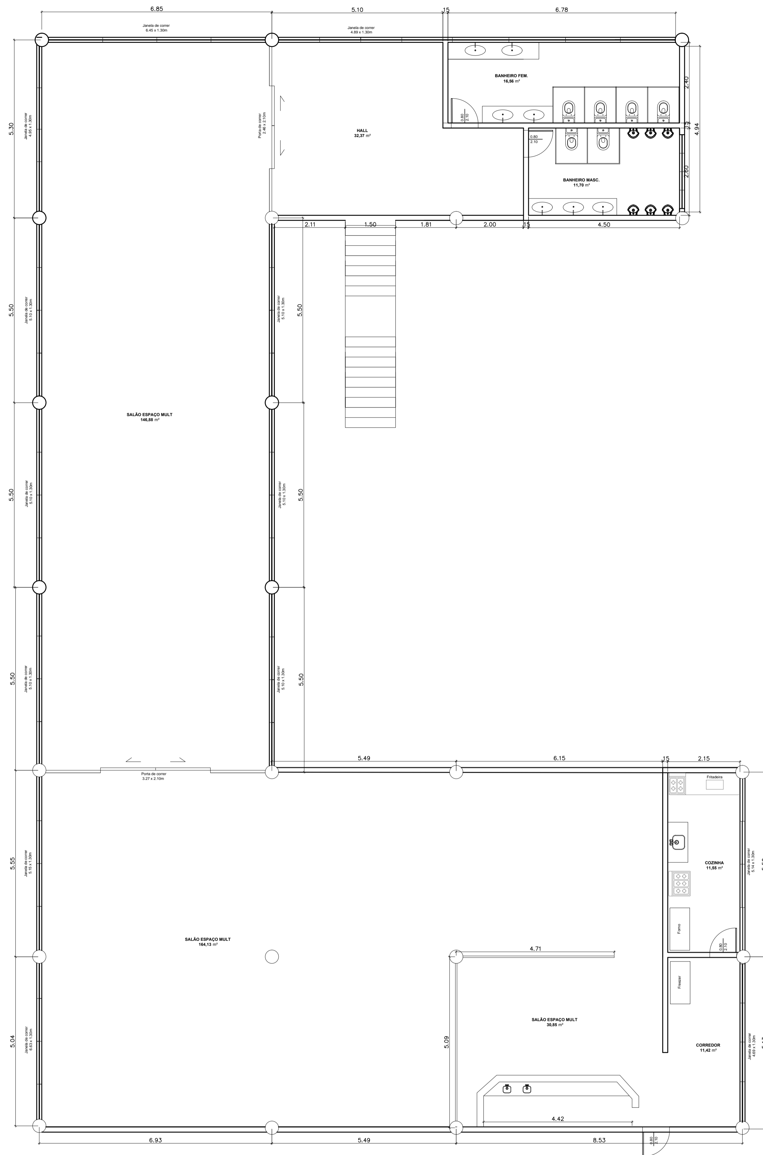
01 Planta Baixa 1/100
